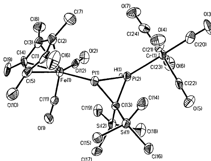
Abb. 1. Molekülstruktur von 9 im Kristall mit ausgewählten Bindungslängen [Å] und -winkeln ^\circ :
